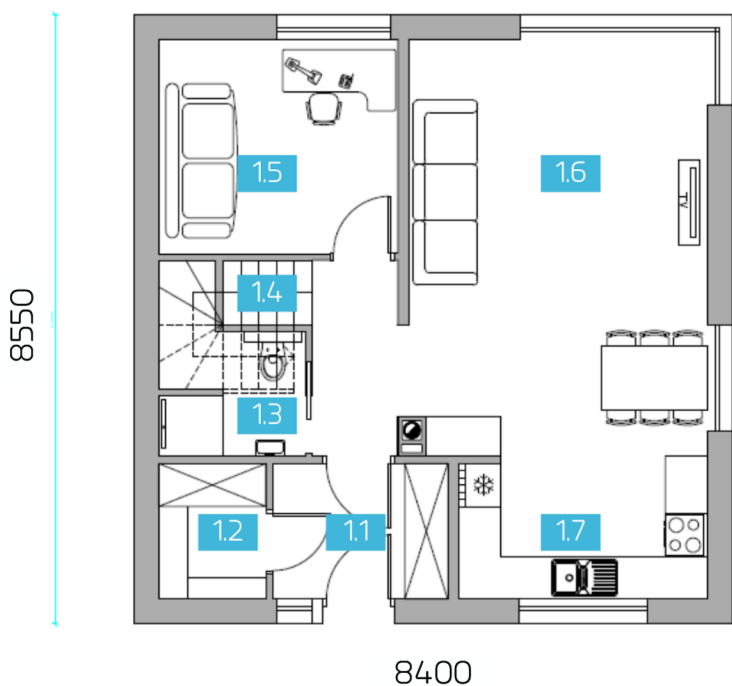
PŘÍZEMÍ
